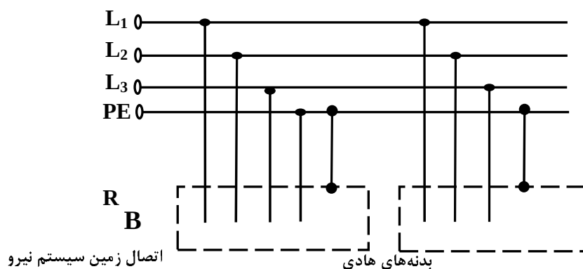
شکل پ ۳ سیستم TN-C با هادی مشترک حفاظتی - خنثی در سرتاسر سیستم.
